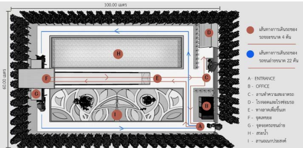
แผนผังแสดงกระบวนการปฏิบัติงานของสถานีขนถ่าย โดยกำหนดกิจกรรมที่สำคัญในการใช้พื้นที่
